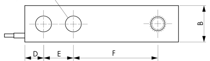
ØG (2 holes)
