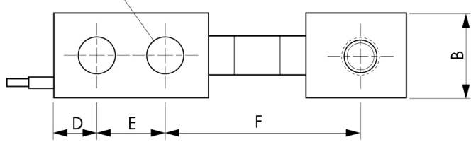
ØG (2 holes)
